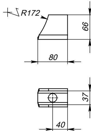
Поз.4 (Ушко)
