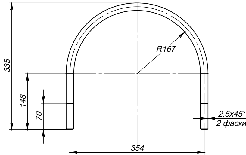
Поз.5 (Хомут)
