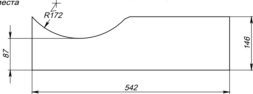
Поз.2 (Угольник)
