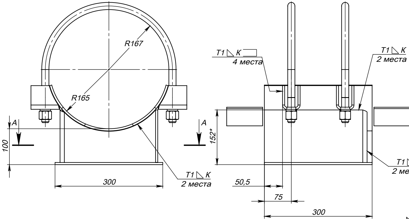
Поз.3 (Ложмент)
