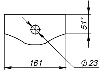
Поз.4 (Ушко) развертка
